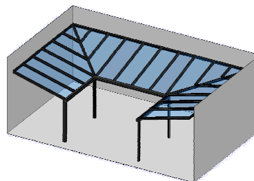
Innenecken
